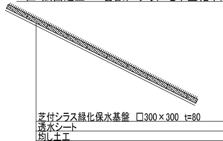
B区: 法面芝生工 害獣(モグラ)・地下茎雑草対策
