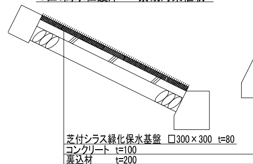
C区: 高水位護岸工 景観対策植栽
